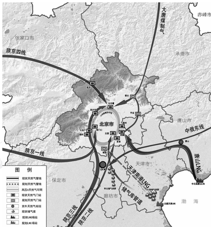
图 5 2025 年北京市天然气设施规划布局示意图
