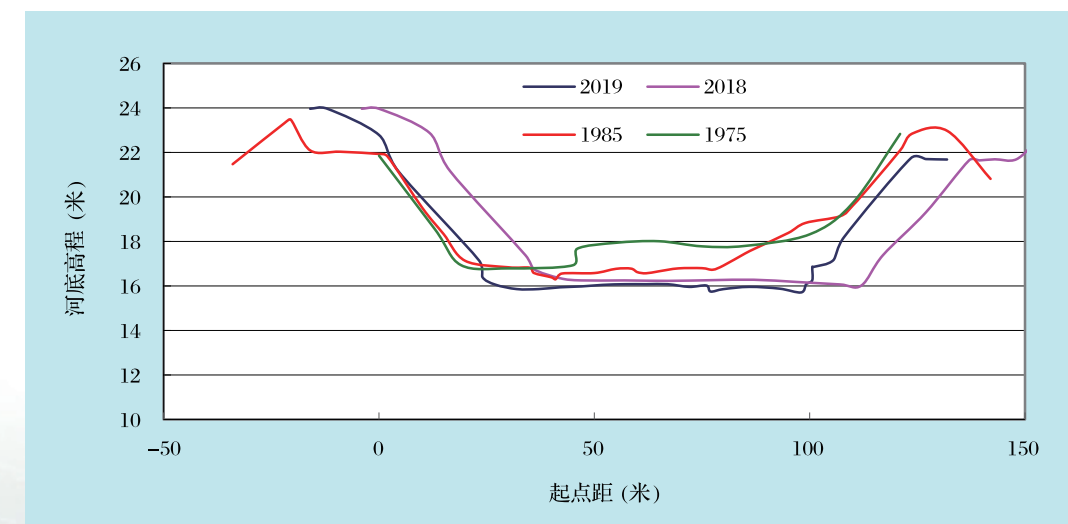
图1-24 运潮减河通县站横断面图
