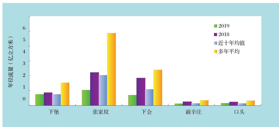
图1-1 潮白河水系各站年径流量对比
