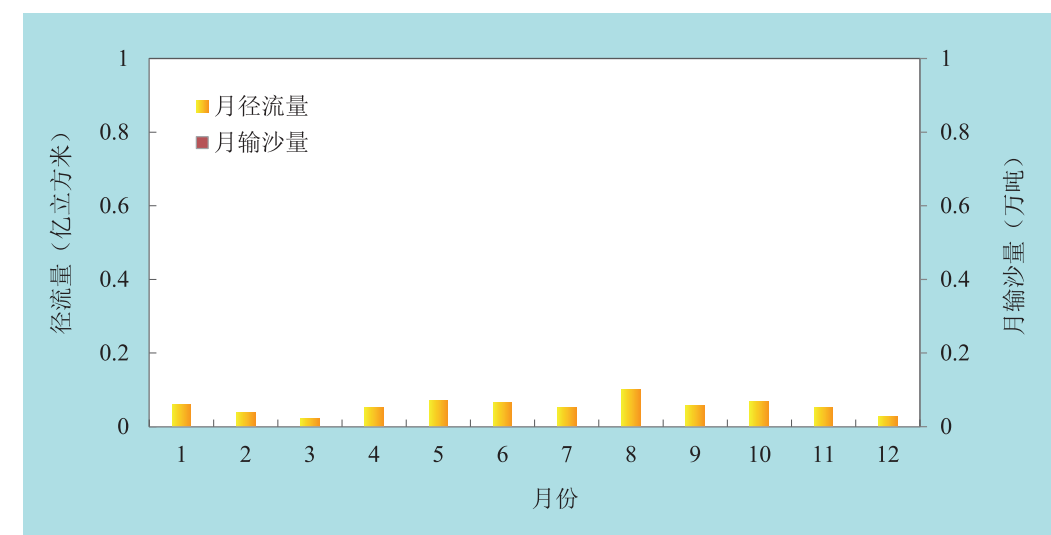
图1-16 张坊水文站2019年逐月径流量与输沙量
