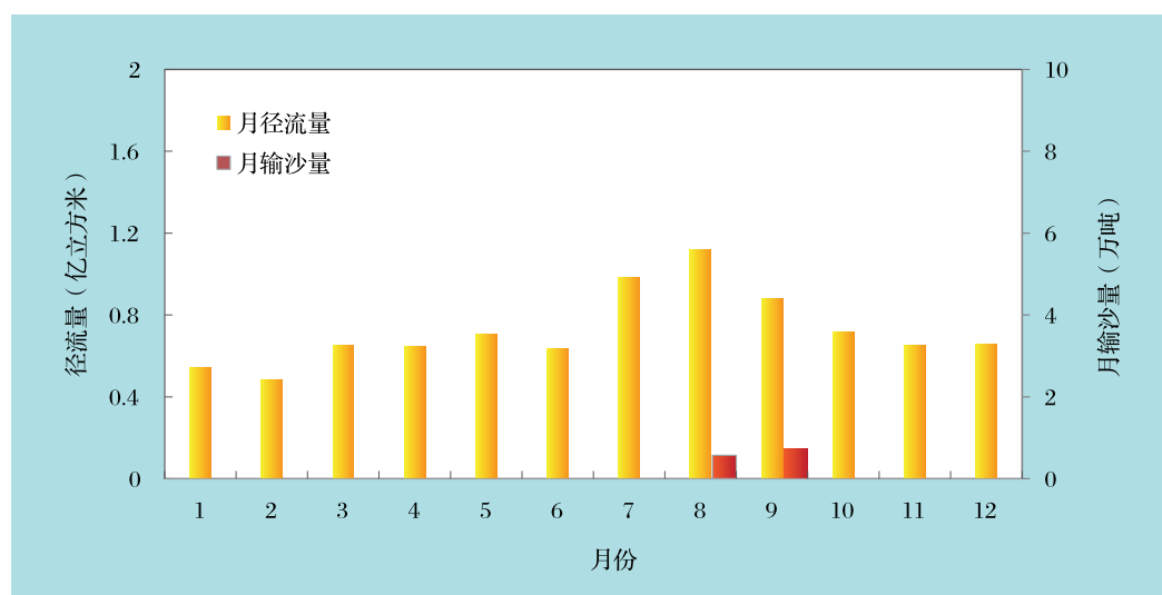
图1-18 通县水文站2019年逐月径流量
