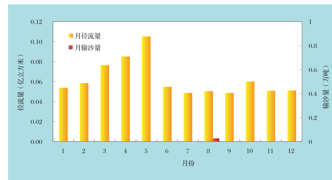
图1-3 下堡水文站2019年逐月径流量
