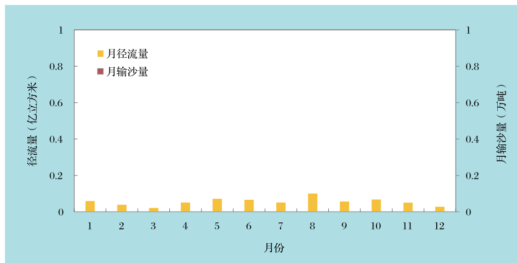
图1-17 漫水河水文站2019年逐月径流量
