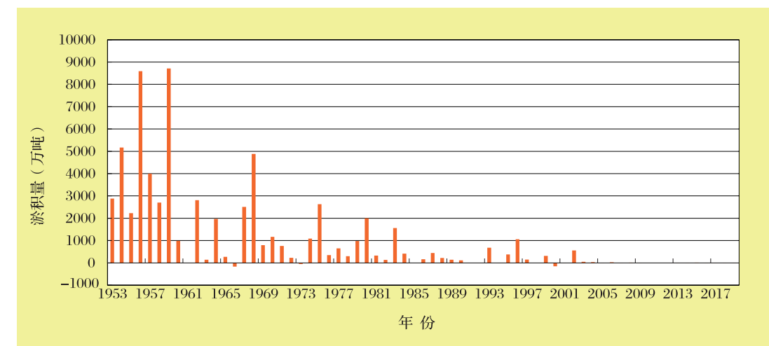
图2-2 官厅水库入库泥沙过程变化图
