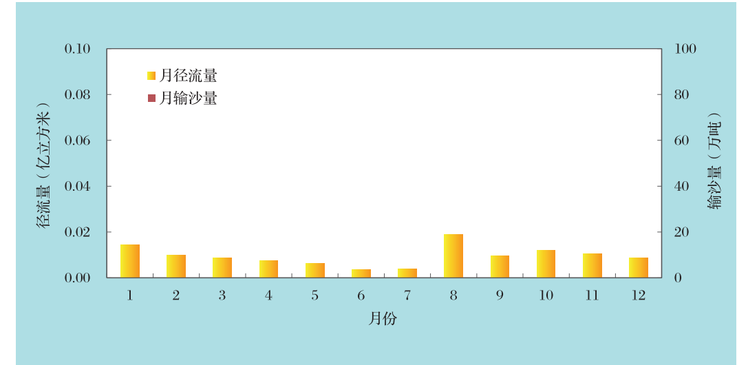
图1-6 前辛庄水文站2019年逐月径流量
