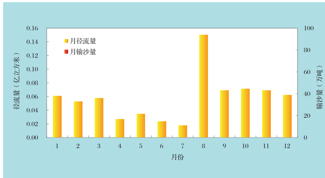
图1-5 下会水文站2019年逐月径流量
