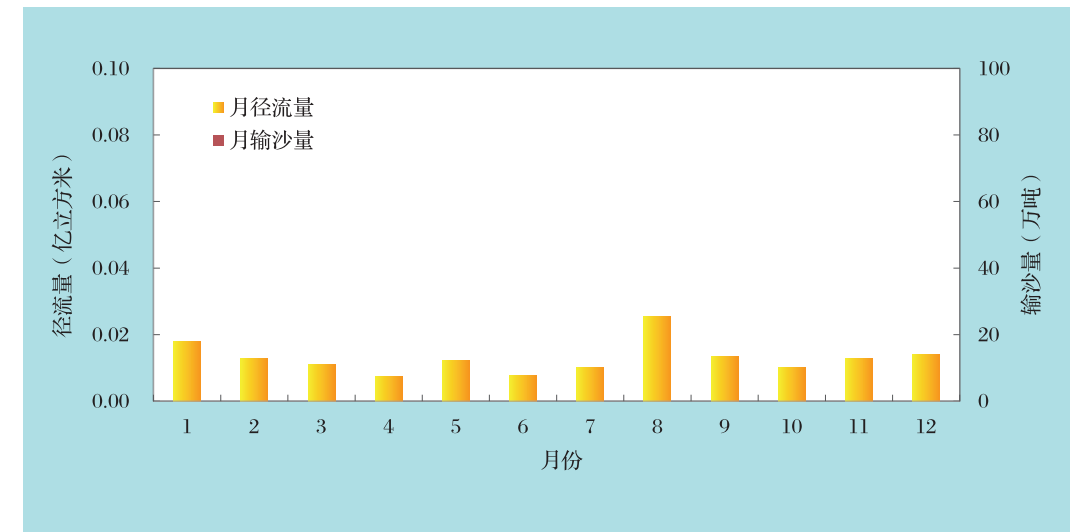
图1-7 口头水文站2019年逐月径流量
