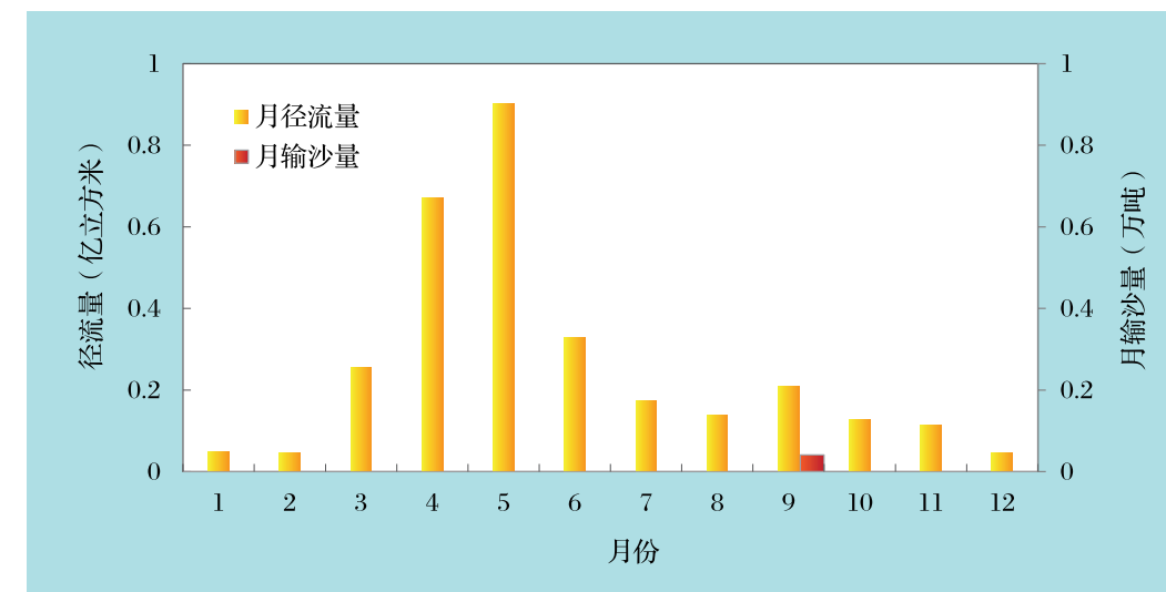
图1-15 雁翅水文站2019年逐月径流量与输沙量
