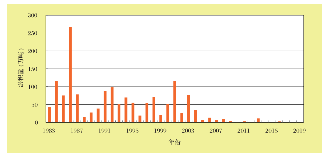
图2-3 白河堡水库入库泥沙过程变化图
