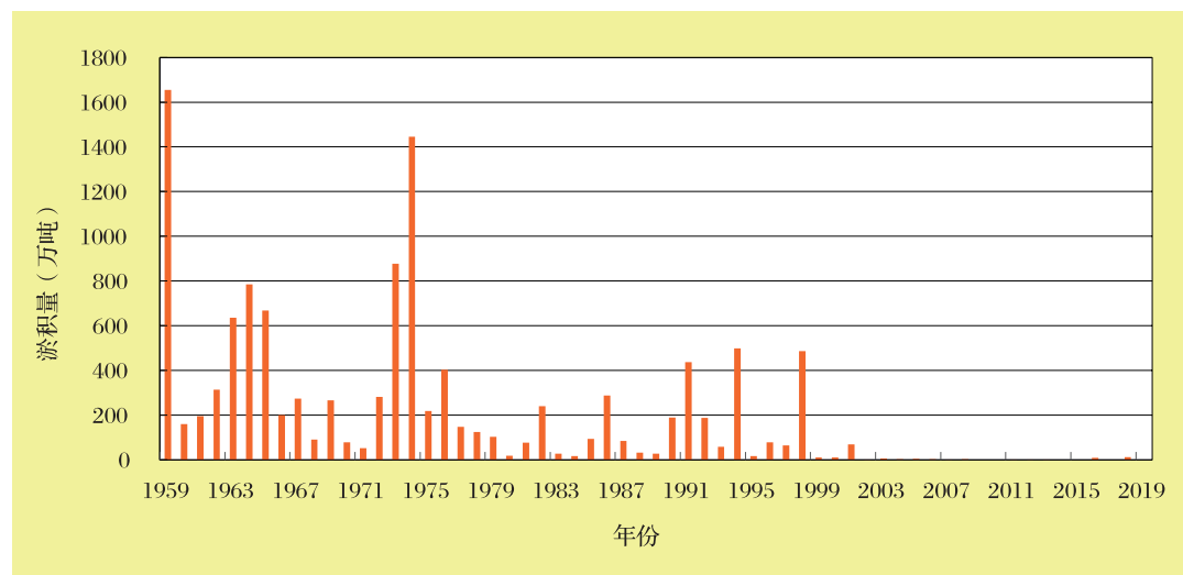
图2-1 密云水库入库泥沙过程变化图
